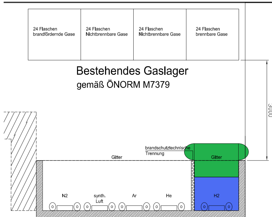
Zentrale Gasversorgungsanlage gemäß ÖNORM M7387-1 lichte Höhe 2,25m
